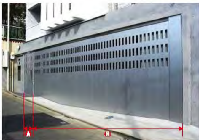
Ⓐ W1,500×H2,000 アルミ製(シルバー) 手動式、片引き仕様、流し込み型 Ⓑ W7,000×H2,500 アルミ製(シルバー) 電動式、片引き仕様、BOX型
